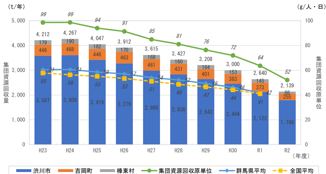
図 3-1-10 集団資源回収量、集団資源回収原単位
