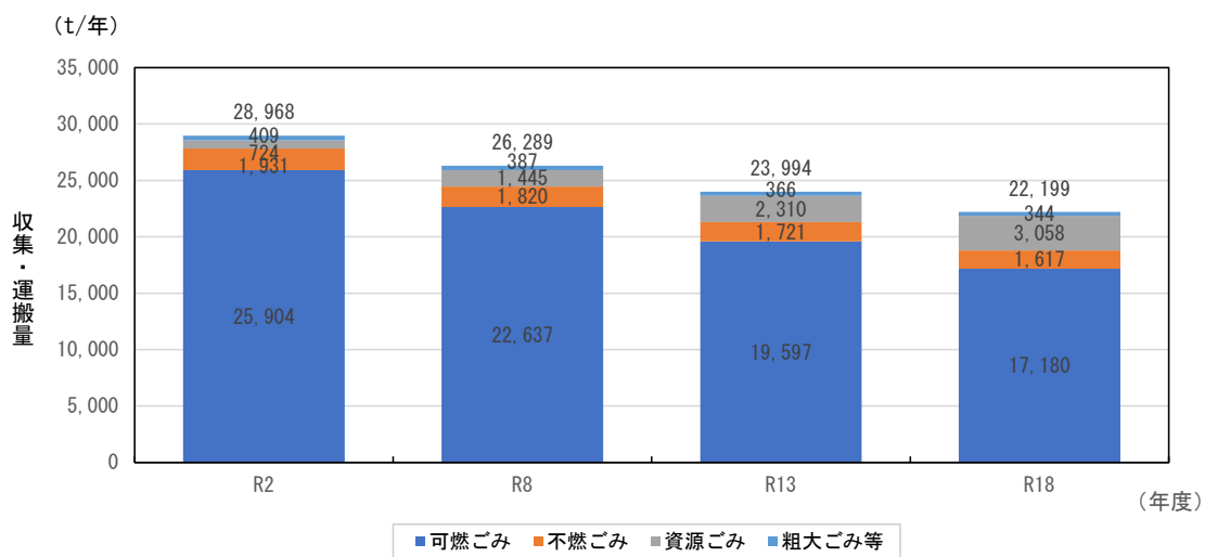
図 3-3-9 収集・運搬量の見込み
