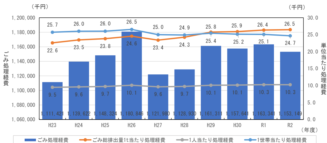
図3-1-26 ごみ処理経費
