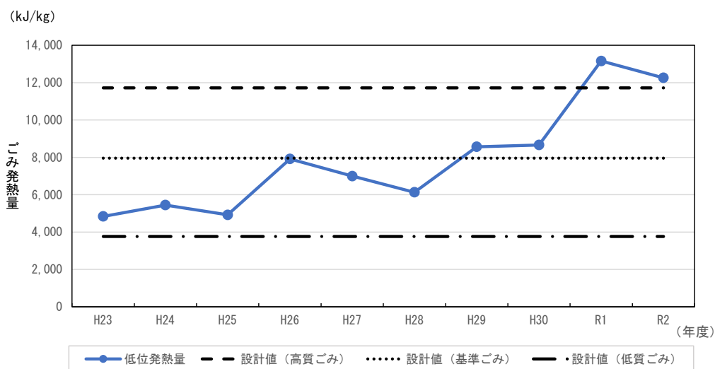
図 3-1-13 ごみ発熱量（低位発熱量）
