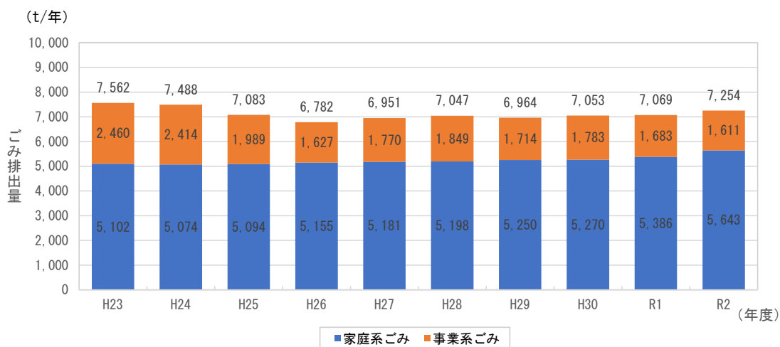
図 3-1-7 ごみ排出量の家庭系ごみ、事業系ごみ（吉岡町）
