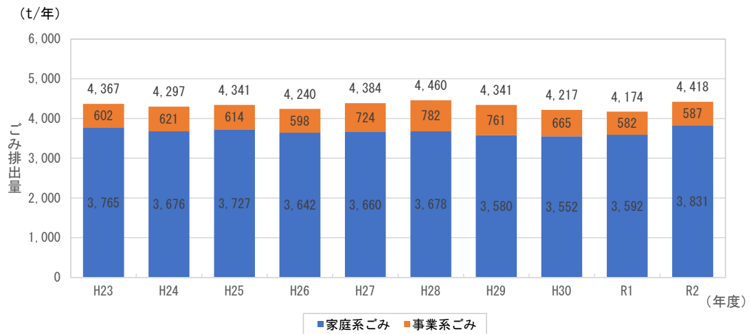
図 3-1-9 ごみ排出量の家庭系ごみ、事業系ごみ（榛東村）
