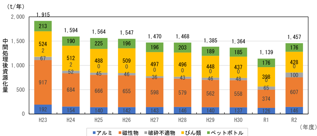
図3-1-23 中間処理後の資源化量
