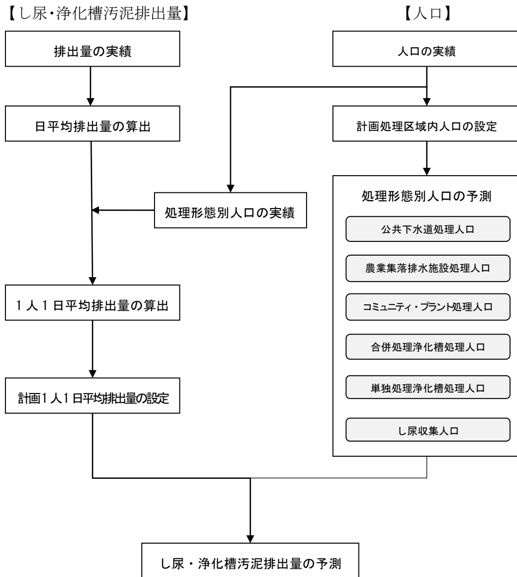
図4-2-1 し尿・浄化槽汚泥量等の予測方法
