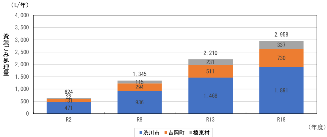
図 3-3-12 資源ごみ処理量の見込み
