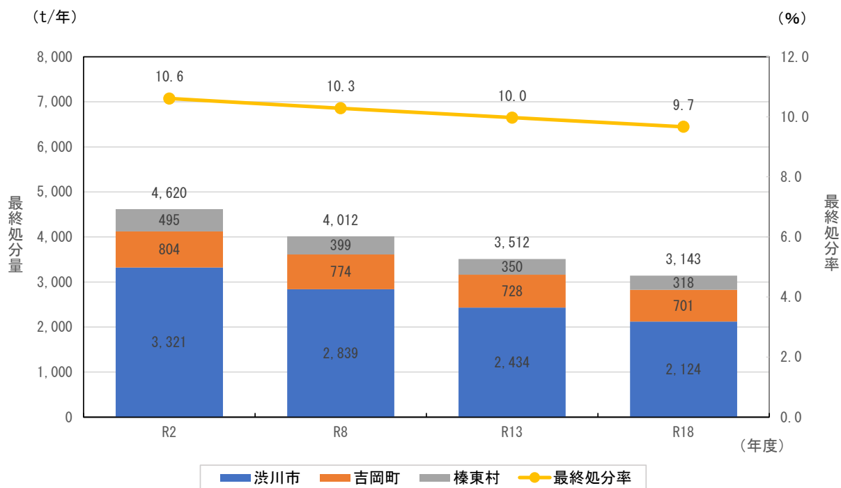
図 3-3-13 最終処分量の見込み
