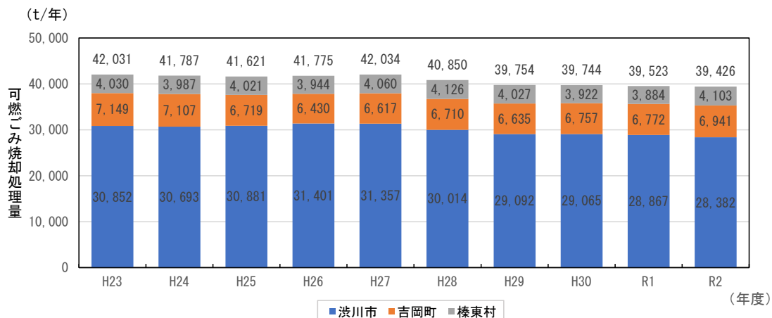
図 3-1-19 可燃ごみ焼却処理量
